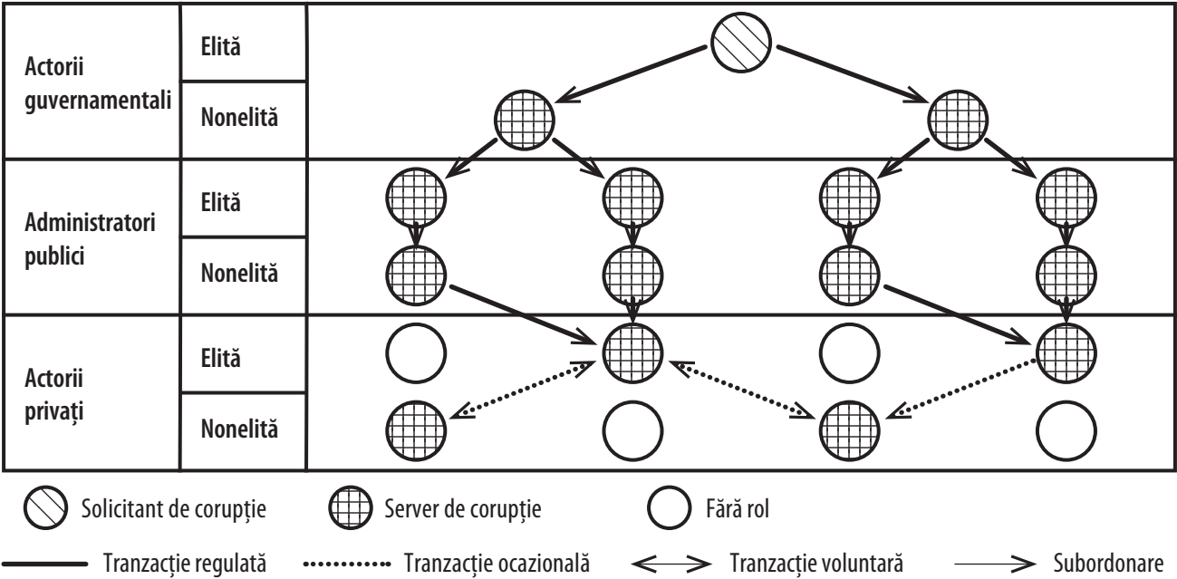
Figura 5.7. Reprezentarea schematică a modelului de stat infrafracțional.
